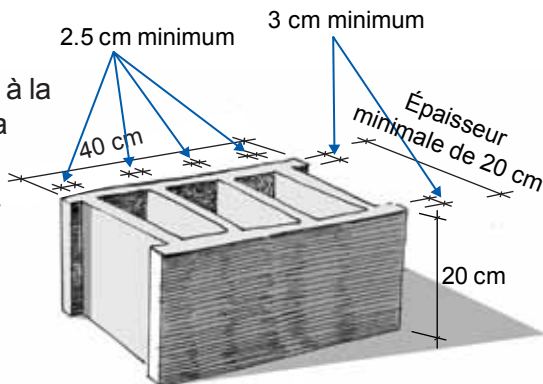
Bloc à trois alvéoles
