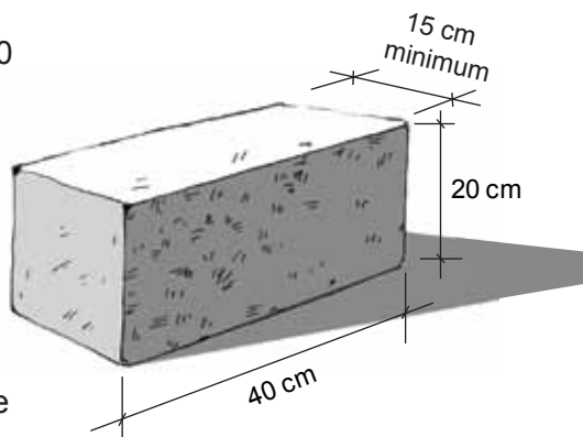
Bloc de béton plein
